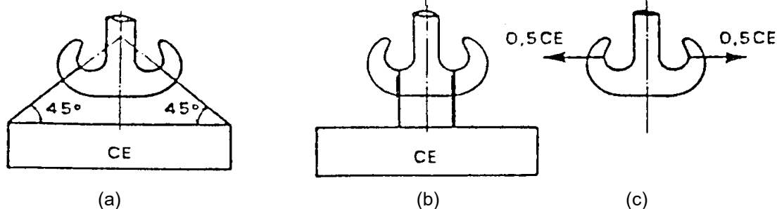
Essai des crochets doubles
